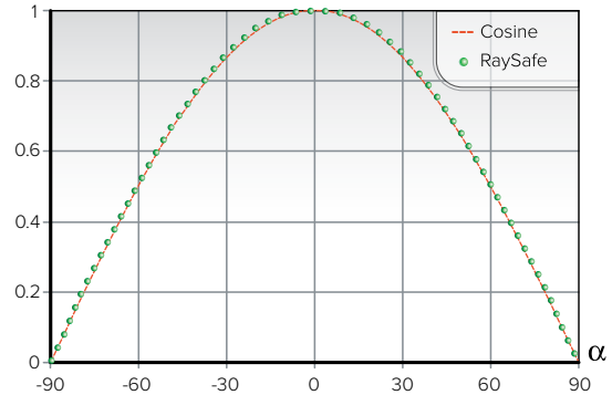
Cosinusanpassung
